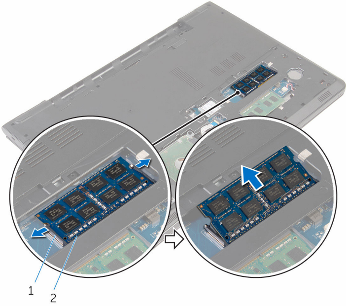
2 内存模块
